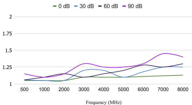
INPUT VSWR
