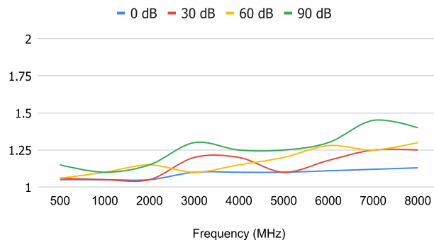
OUTPUT VSWR
