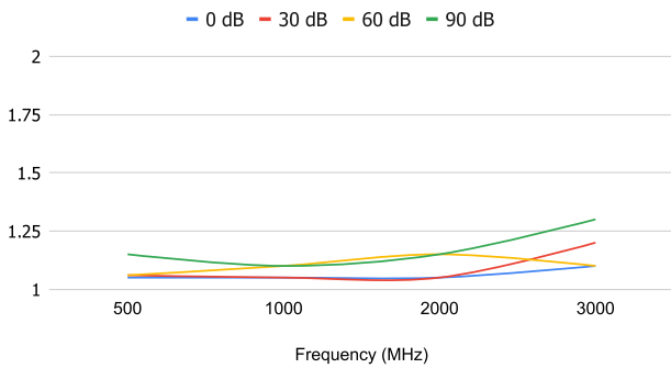
OUTPUT VSWR
