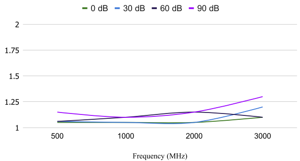
INPUT VSWR
