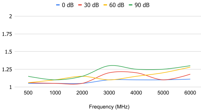
OUTPUT VSWR
