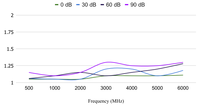
INPUT VSWR
